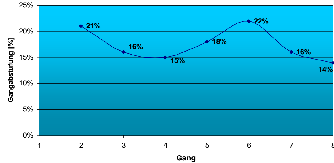
Gangabstufung Nexus 8
