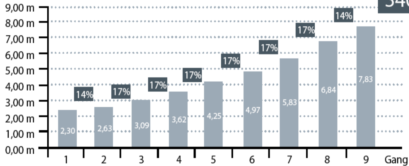
Zurückgelegte Wegstrecke pro Kurbelumdrehung (m) bei 38/20
