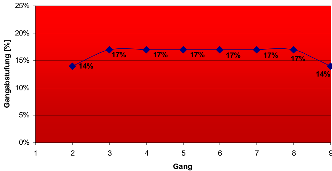
Gangabstufung i-MOTION 9
